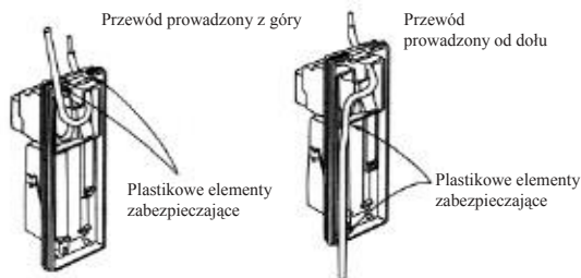
Przewód prowadzony z góry
